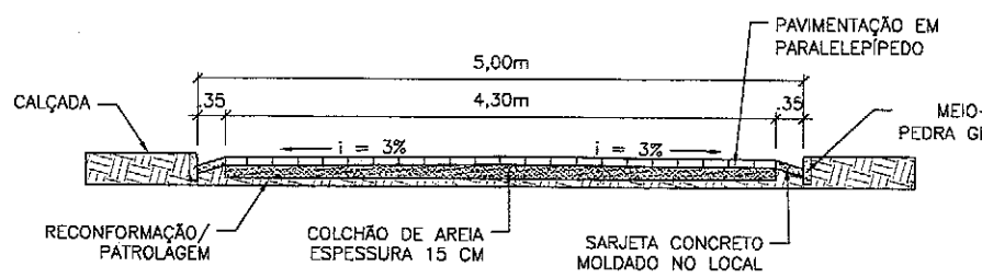
DETALHE SEÇÃO TRANSVERSAL - TRECHO (ESTACA 00 À 01+9.60M) ESCALA 1:50
