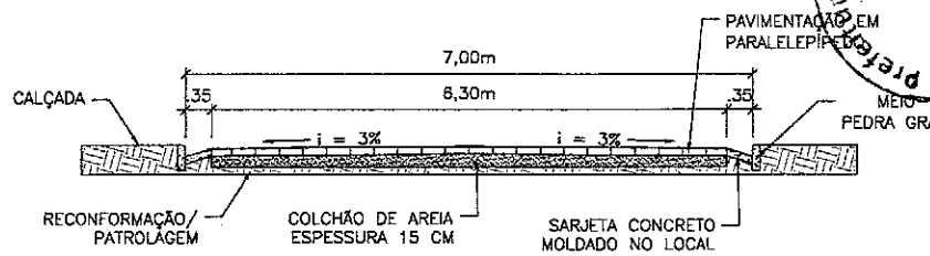
DETALHE SEÇÃO TRANSVERSAL - TRECHO (ESTACA 02+2.55M À 04+17.33M) ESCALA 1:50
