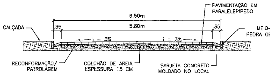
DETALHE SEÇÃO TRANSVERSAL - TRECHO (ESTACA 01+9.59M À 02+2.65M) ESCALA 1:50
