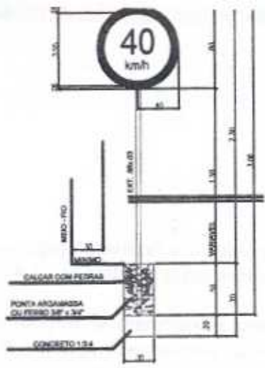
DETALHE DA SEÇÃO SINALIZAÇÃO ESCALA _____ 1/ESCALA _____
