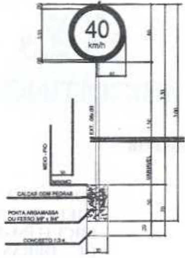
○ DETALHE DA SEÇÃO SINALIZAÇÃO ESCALA _____ DESCALA _____
